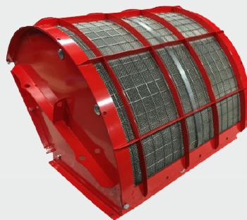
Flamefree™ 爆発放散口
