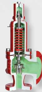
バックリングピン式 リリーフバルブ
